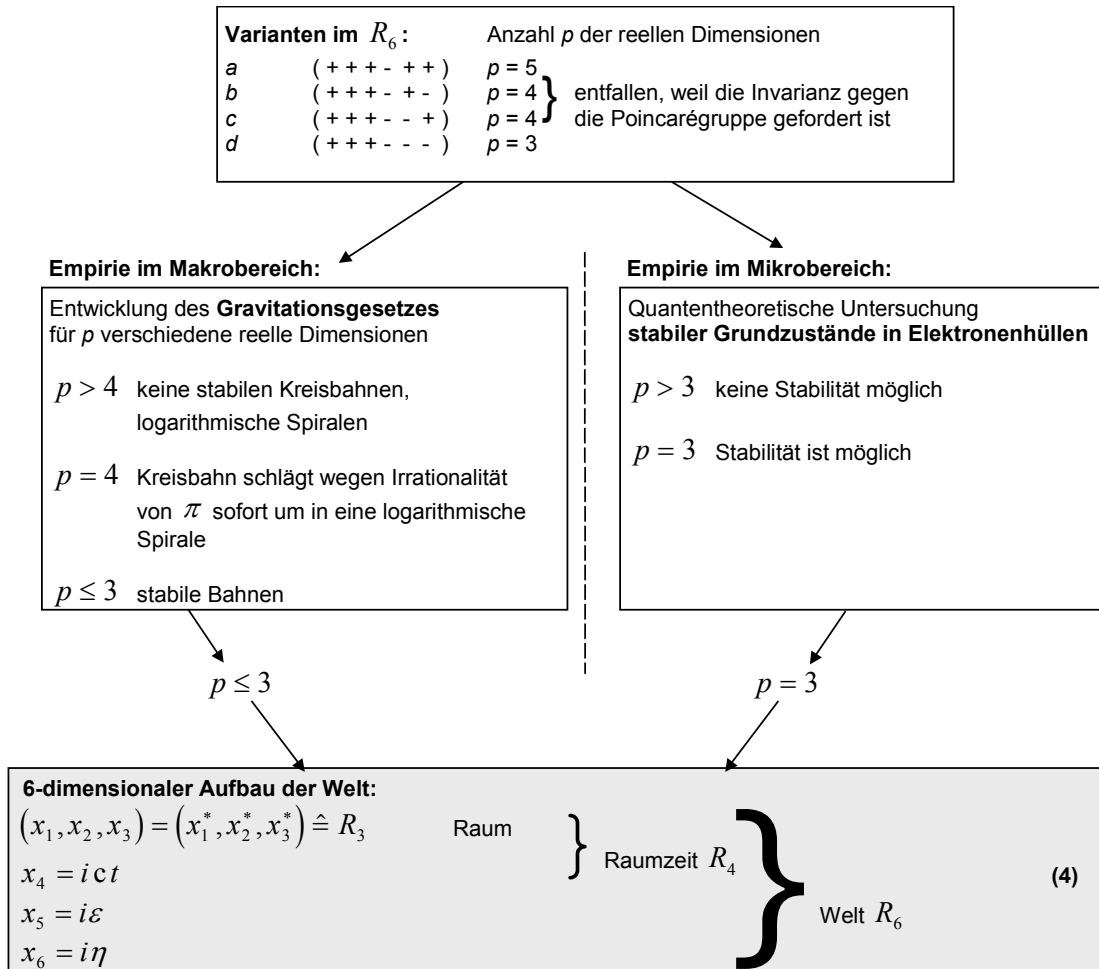
Abbildung 9: Bestimmung des algebraischen Charakters der Dimensionen x_5, x_6
