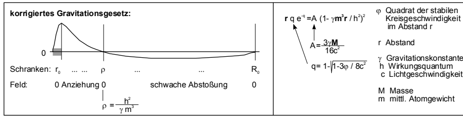
Abbildung 10: Qualitativer Verlauf des korrigierten Gravitationsgesetzes ( \frac{d\phi}{dr} )
