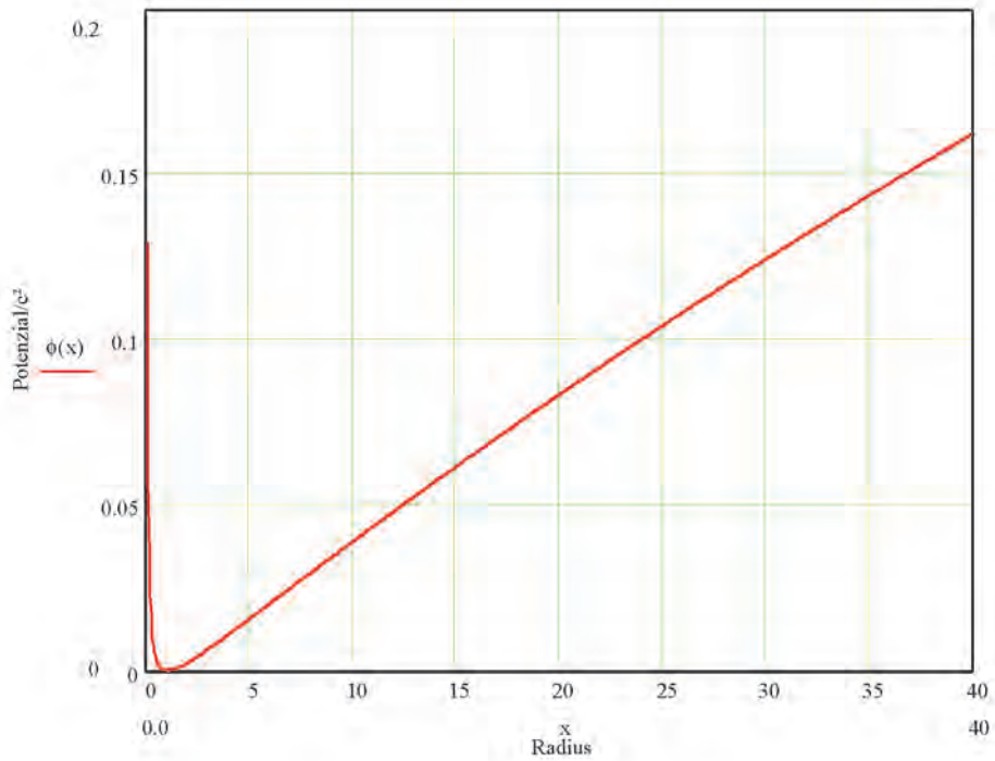
Abbildung 5: Grundsätzlicher Verlauf des Heimschen Gravitationspotenzials im Fall \beta > 0
