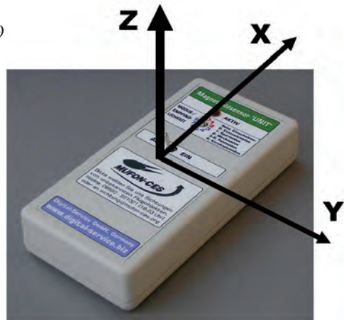
Bild 1: Magnetfeldkomponenten
