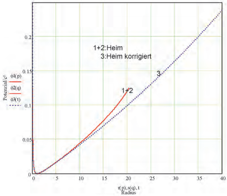
Abbildung 2: Grundsätzlicher Verlauf des Heimschen Gravitationspotenzials
