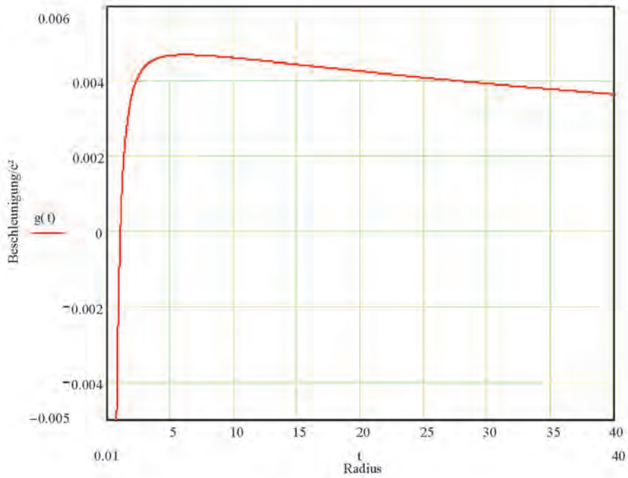
Abbildung 4: Ortsabhängigkeit der Beschleunigungsfunktion im Fall \beta > 0
